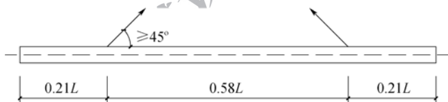
图 7.2.2-1 长度不大于 15m 的预应力混凝土桩吊点位置
