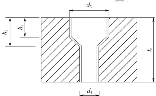
图 6.2.15 端板锚固孔示意图
