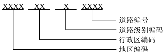
图 4.2.2 地下市政基础设施普查单元编号结构图
