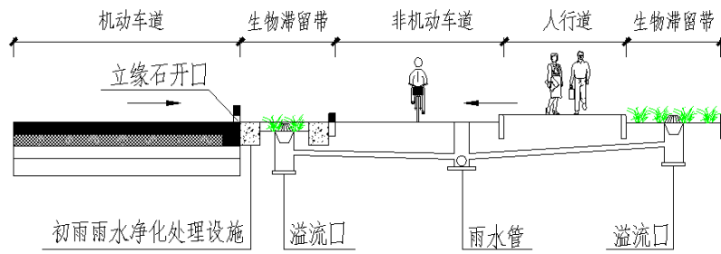
典型道路系统断面图
