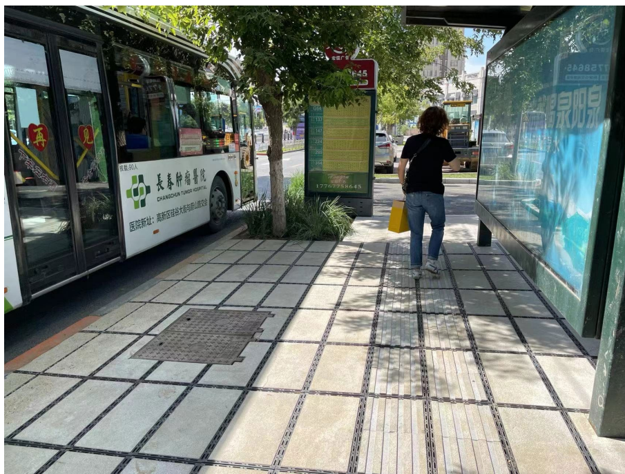
图 4-4 渗排板与仿石材缝隙型透水砖/花岗岩组合铺装示意图
