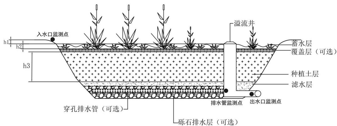
图 9-2 生物滞留设施结构与监测点位布置示意图
