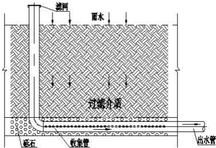
图 8-14 介质过滤设施示意图
