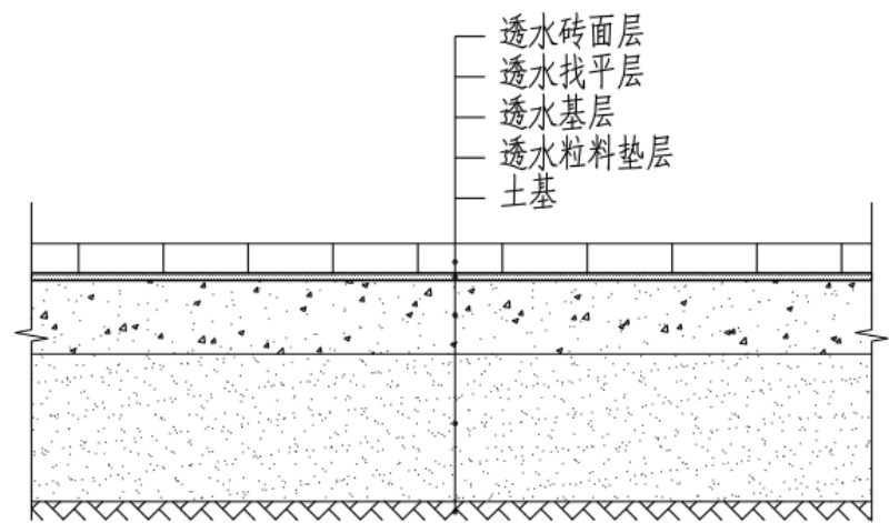
透水砖铺装基本构造
