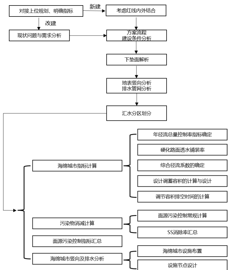
图 5-2 城市道路海绵城市设计与计算流程示意图
