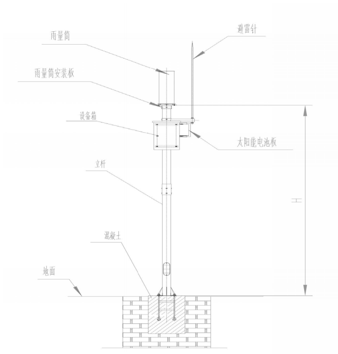
图 9-7 翻斗式雨量计安装示意图
