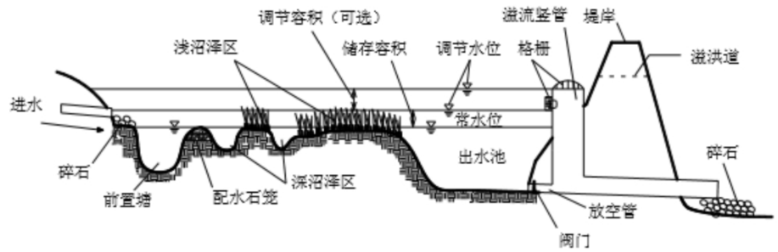
图 8-8 雨水湿地典型构造示意图
