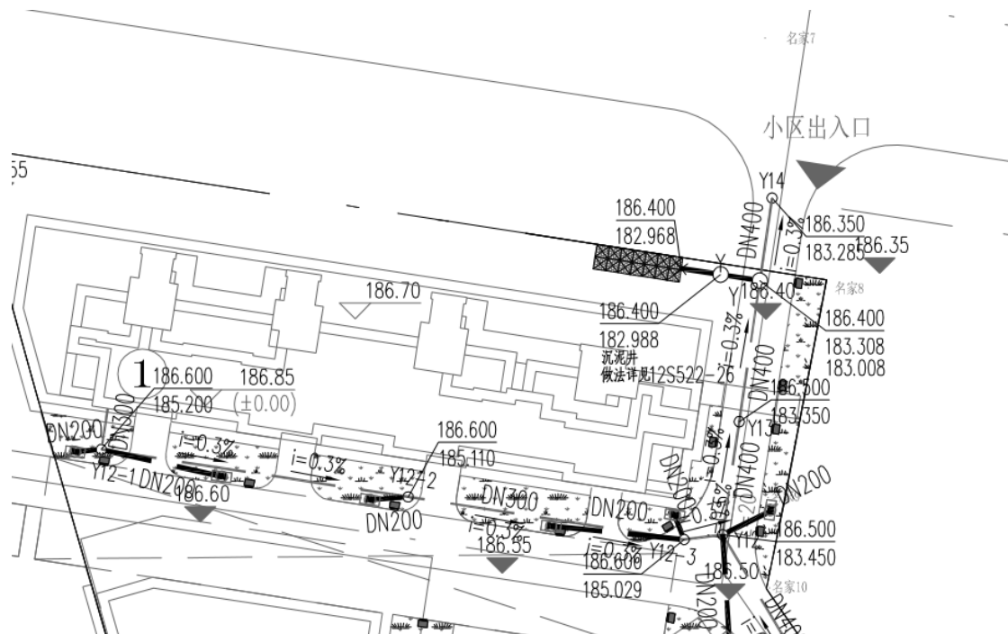
图 10-6 海绵城市设施雨水管网图
