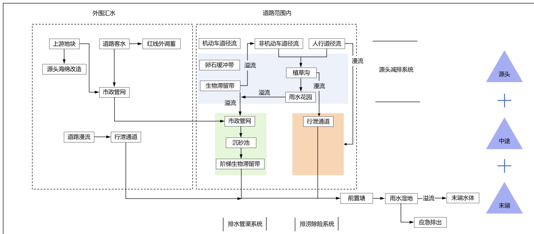
图 5-1 典型海绵型道路雨水径流组织技术路线
