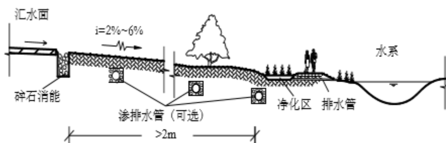
图 8-12 植被缓冲带典型构造示意图
