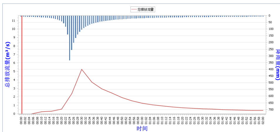
图 10-32 50 年一遇 2h 降雨量与总排放量对比图
