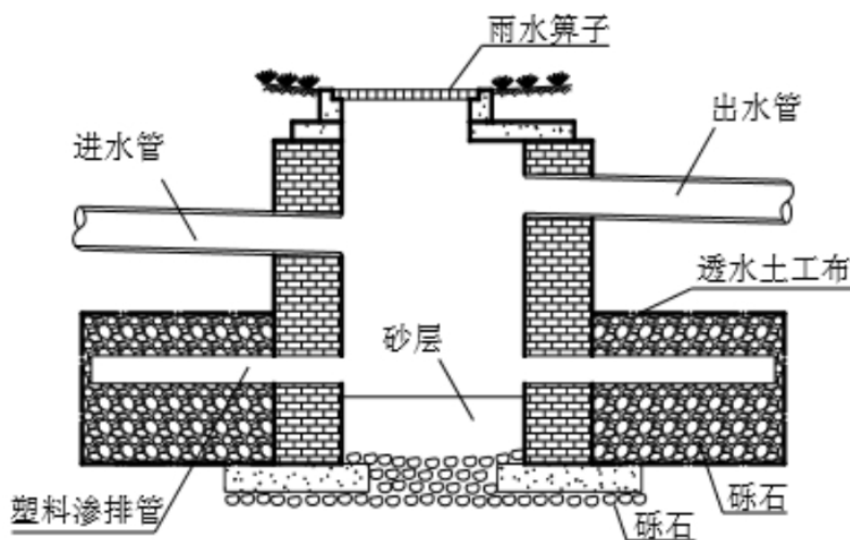
图 8-6 辐射渗井构造示意图
