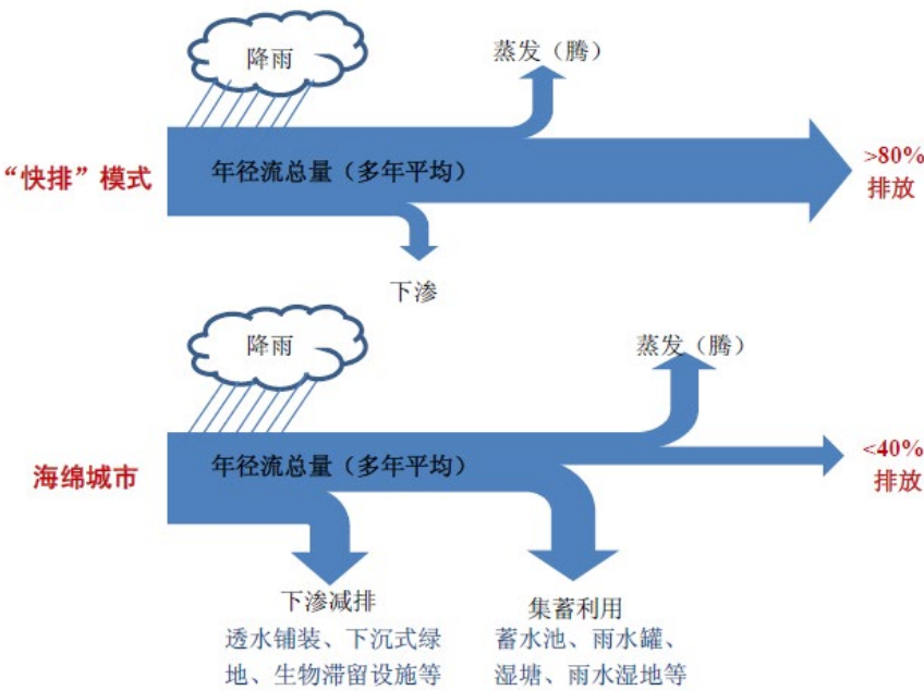
图 10-24 年径流总量控制率概念示意图
